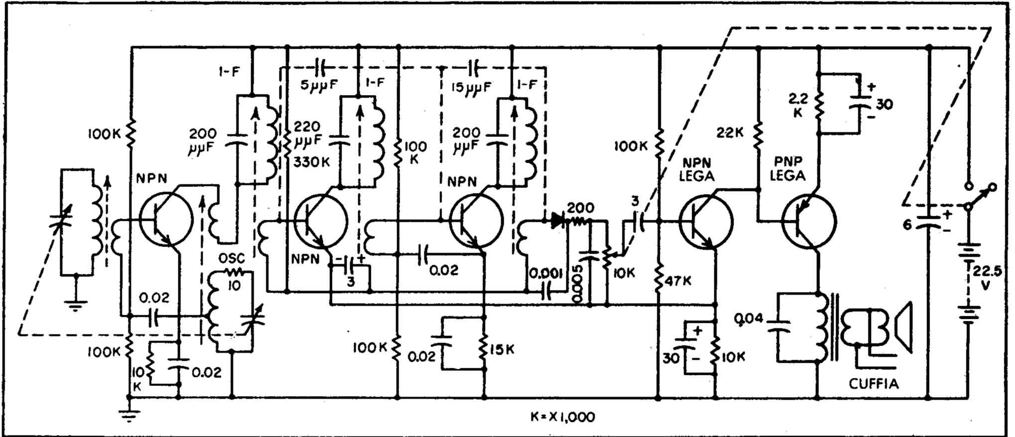
SCHEMA ELETTRICO DEL RADIORICEVITORE « SONY TR-57 » DELLA TOKYO TSUSHIN KOGYO, Ltd.
